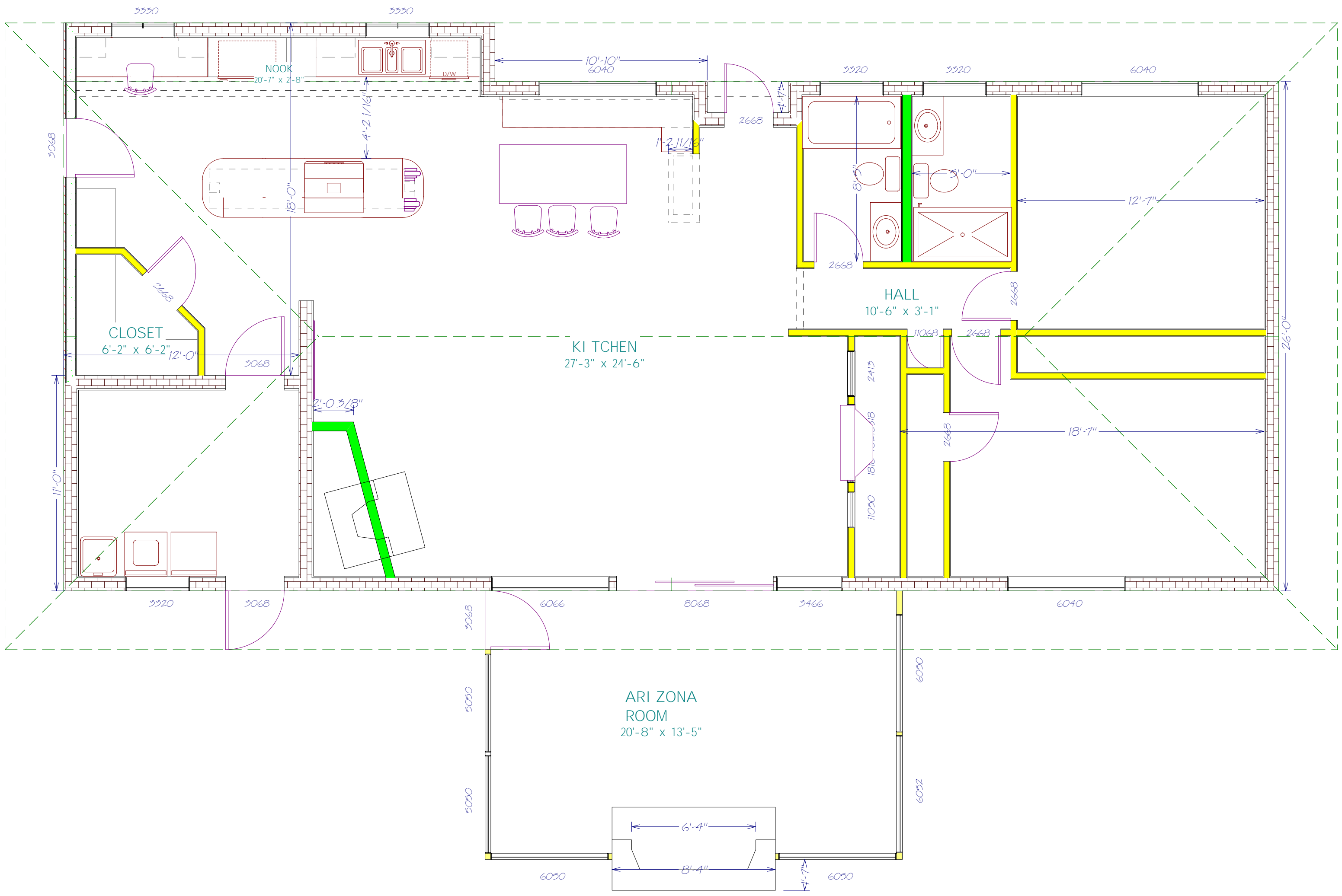
LI VI NG AREA 1967 sq ft
